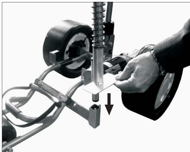
5. Introducir en el cuadradillo del soporte base la parte superior del asiento.
