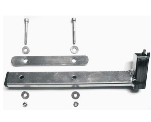
2. Detalle de colocación de tornillos y arandelas en el soporte base.
